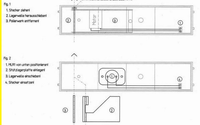
Montageplan für MLR-1 Art.-Nr. 9124 oder 9031
